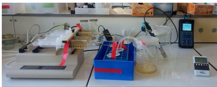
Figure 3.3 – Système d'alimentation pousse-seringue multicanaux
