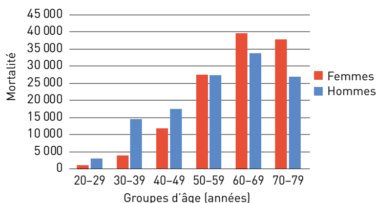
Figure 4.5.2 Mortalité due au diabète par âge et par sexe, Région Amérique Centrale et du Sud, 2019
